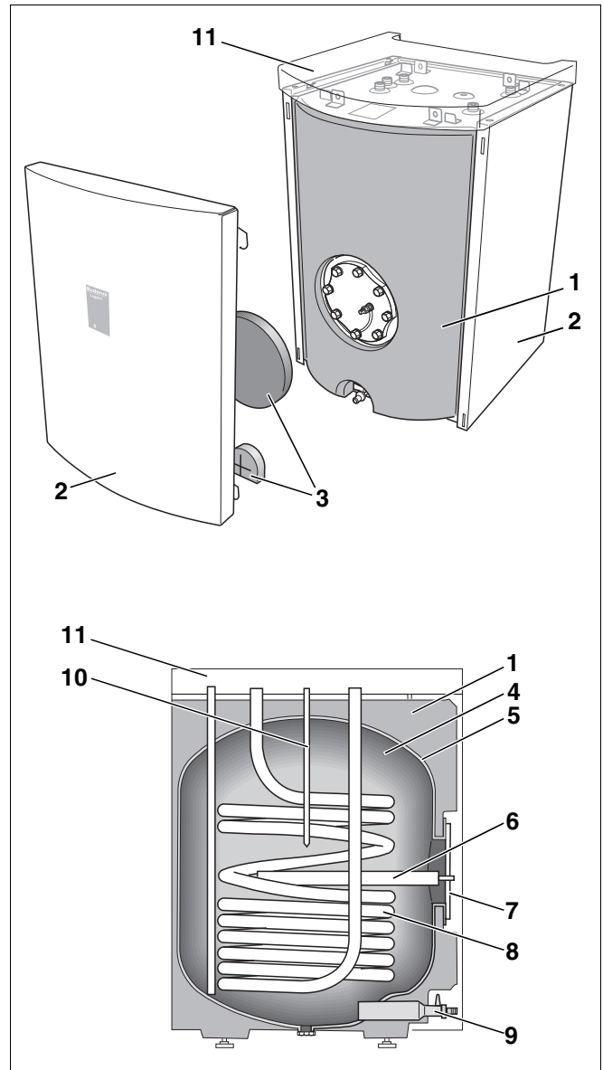
Abb. 1 Warmwasserspeicher Logalux S135/S160 (unten schematische Darstellung)
