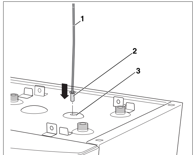
Abb. 10 Temperaturfühler montieren
