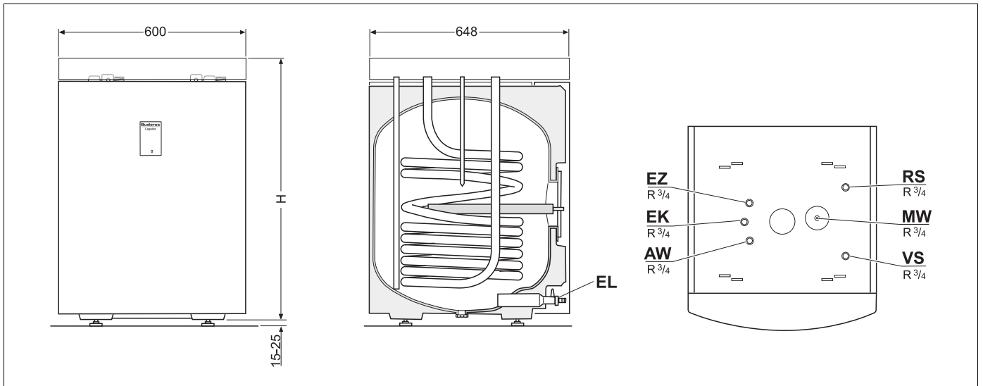
Abb. 2 Abmessungen und Anschlüsse (Maße in mm)
