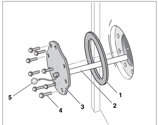
Abb. 17 Magnesiumanode einbauen
