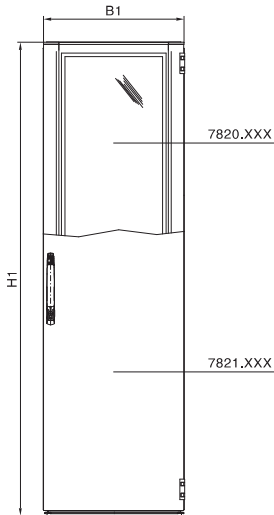
Vorderansicht
