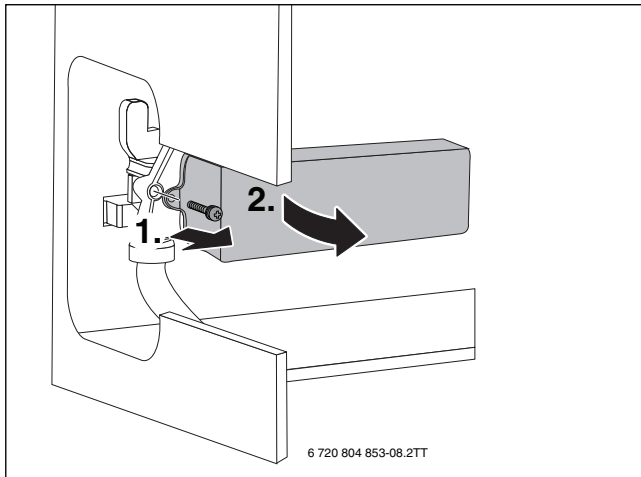
Bild 57 Plattenwärmetauscher ausbauen
