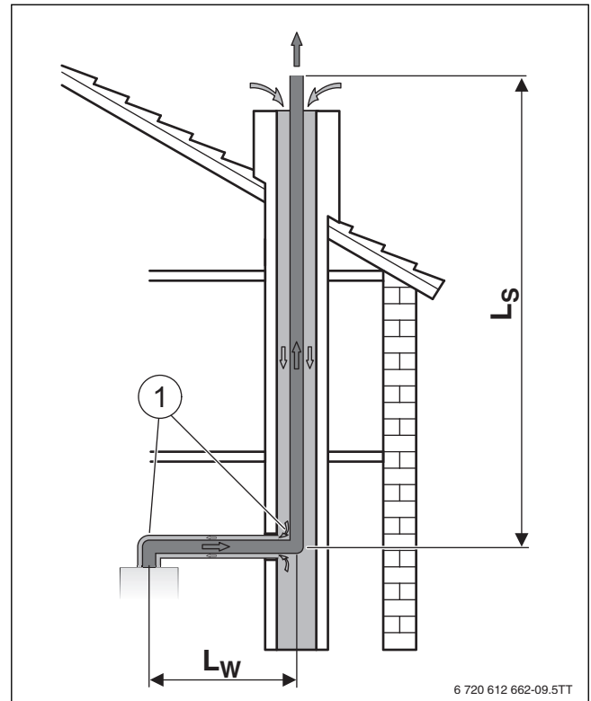
Bild 14 Abgasführung im Schacht nach C 93x
