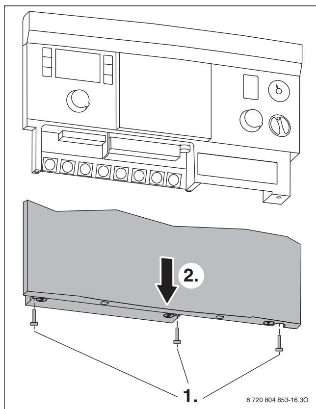
Bild 29 Abdeckung entfernen
