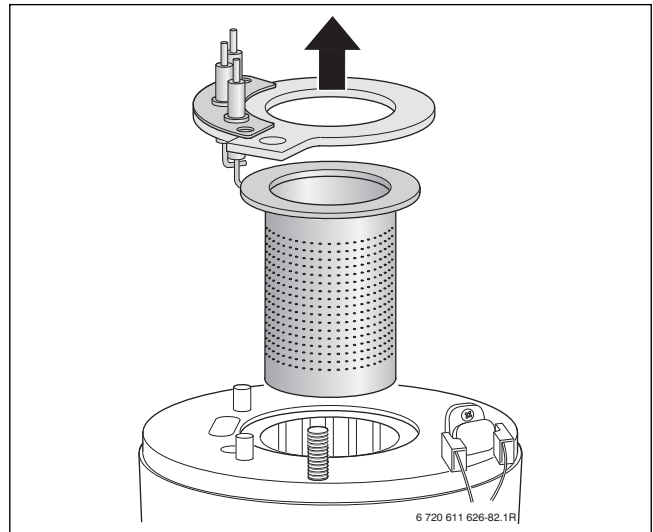
Bild 47 Brenner herausnehmen
