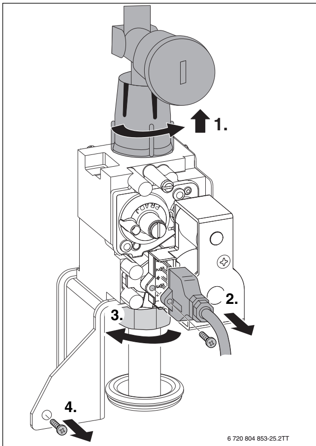
Bild 62 Gasarmatur ausbauen
