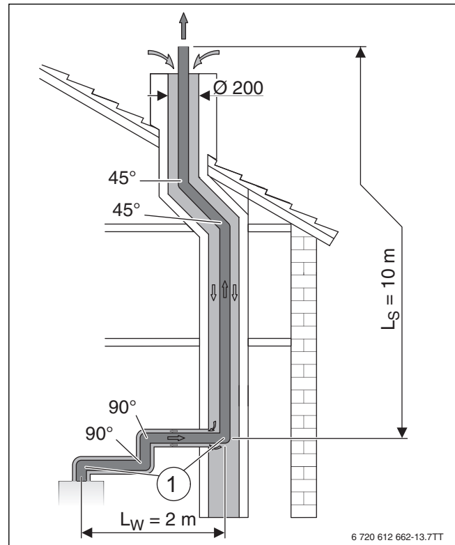
Bild 20 Einbausituation einer Abgasführung nach C 93x
