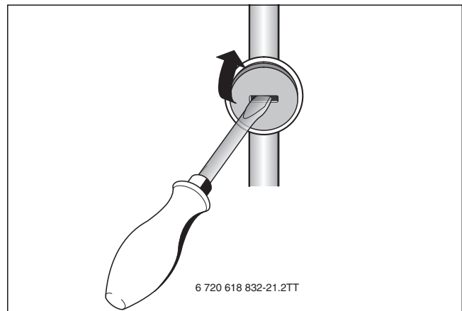
Bild 37 Plombe entfernen
