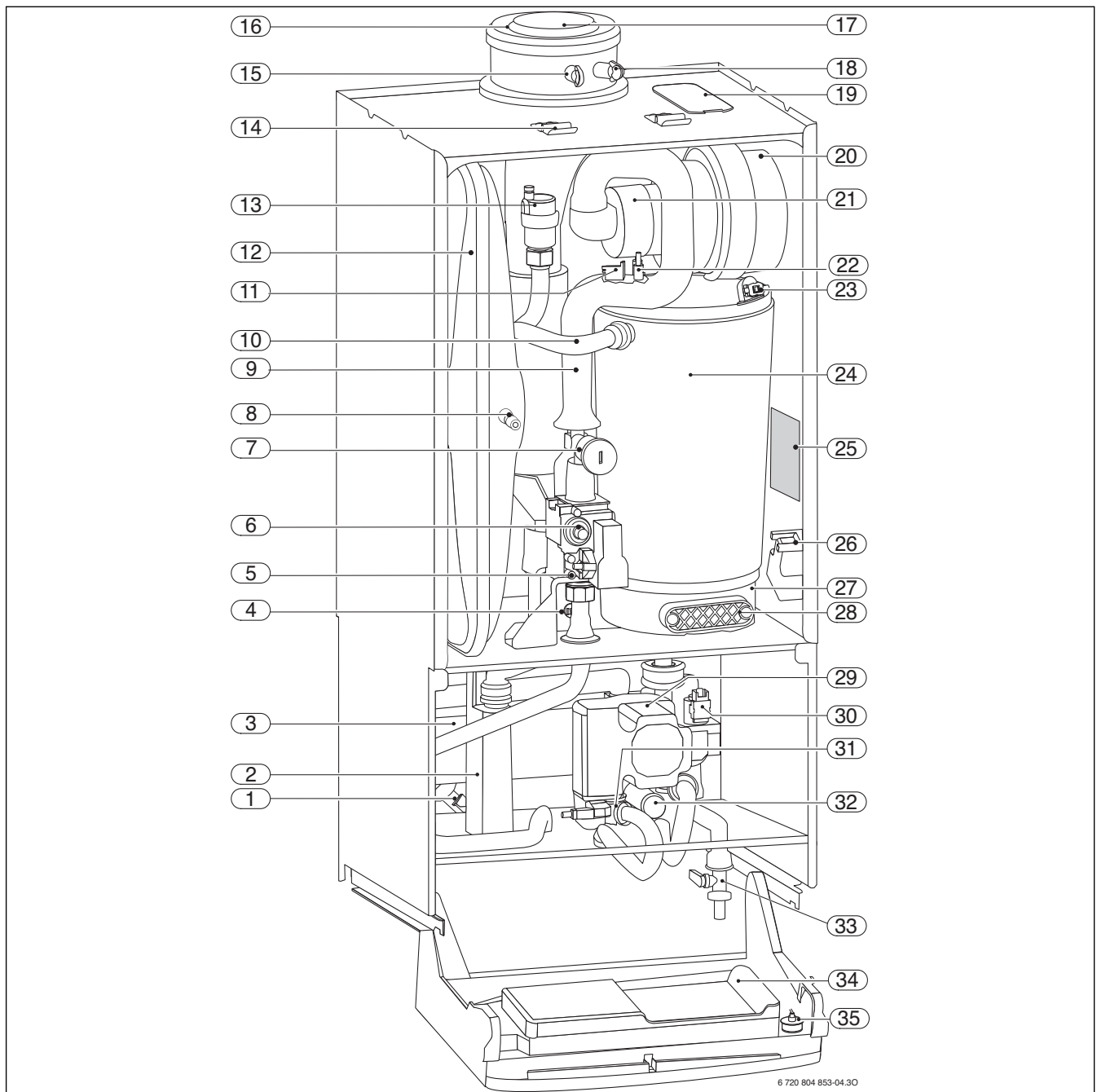
Bild 3 Produktübersicht
