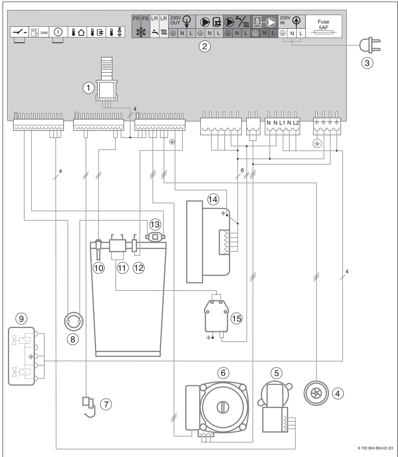
Bild 4 Elektrische Verdrahtung
