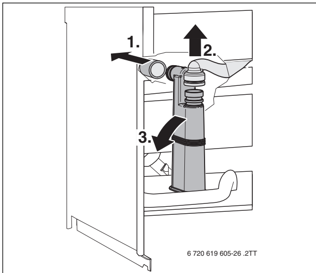
Bild 53 Kondensatsiphon ausbauen
