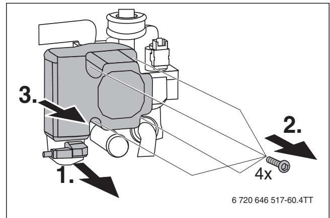
Bild 64 Heizungspumpe ausbauen
