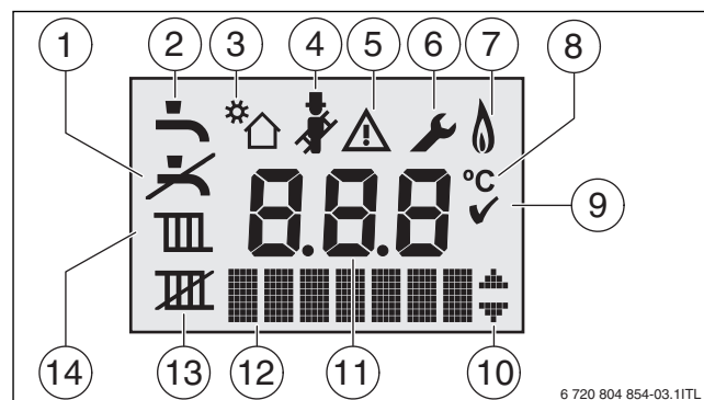
Bild 33 Displayanzeigen
