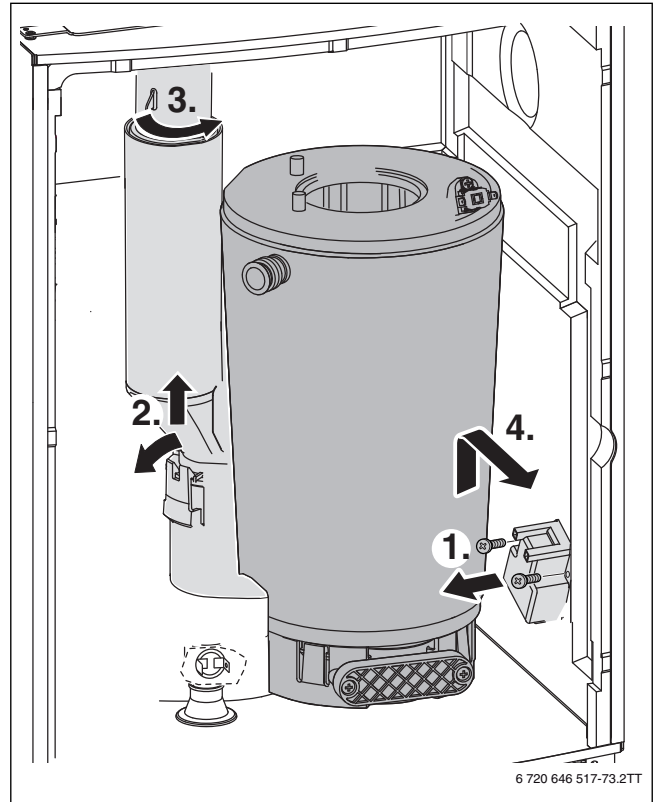
Bild 71 Wärmeblock ausbauen
