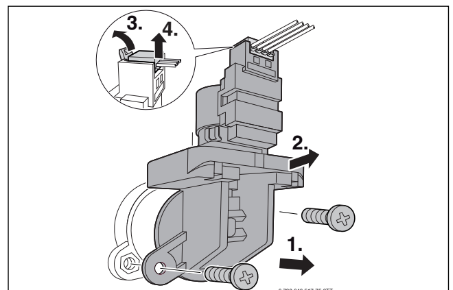
Bild 60 3-Wege-Ventil ausbauen
