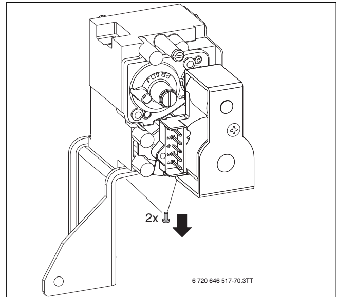
Bild 63 Gasarmatur ausbauen
