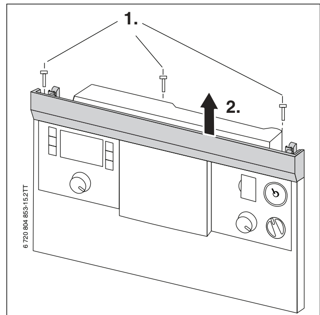
Bild 27 Abdeckung entfernen
