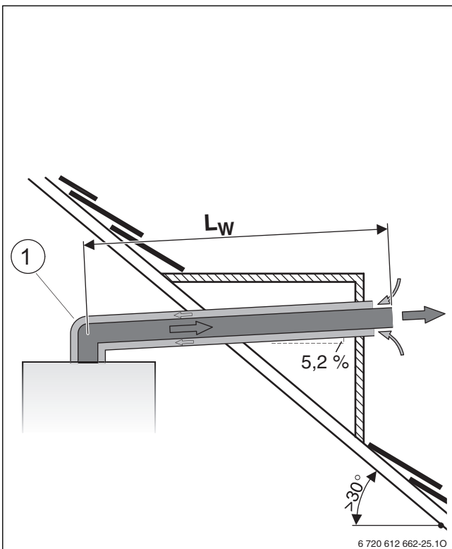
Bild 17 Abgasführung waagrecht nach C 33x (Ø 80/125 mm)
