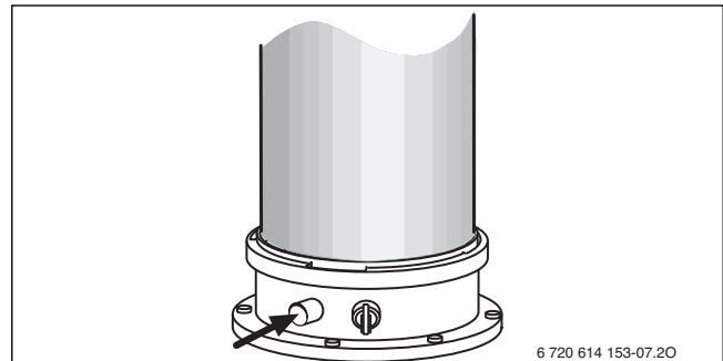
Bild 35 Abgasmessstutzen
