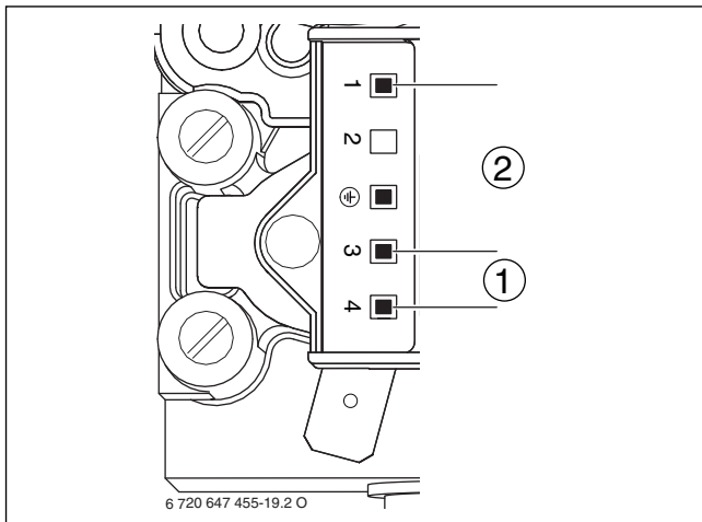
Bild 61 Messstellen an der Gasarmatur
