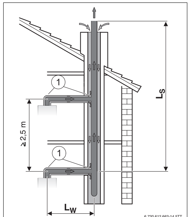
Bild 19 Mehrfachbelegung mit konzentrischem Rohr nach C 43x
