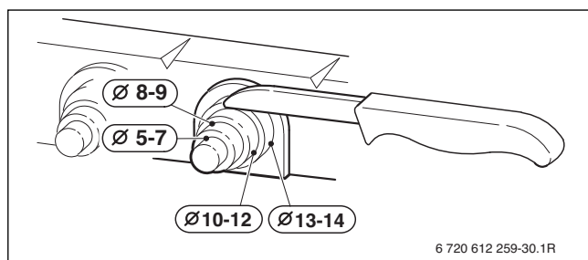
Bild 30 Zugentlastung an Kabeldurchmesser anpassen
