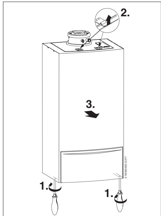
Bild 22 Verkleidung abnehmen
